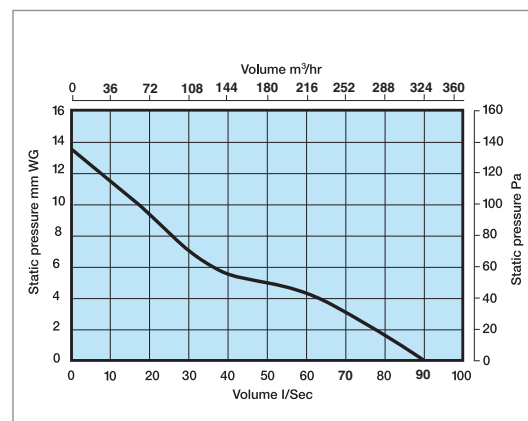
► Performance - EL150
