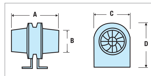
► Dimensions - EL150 Fan
