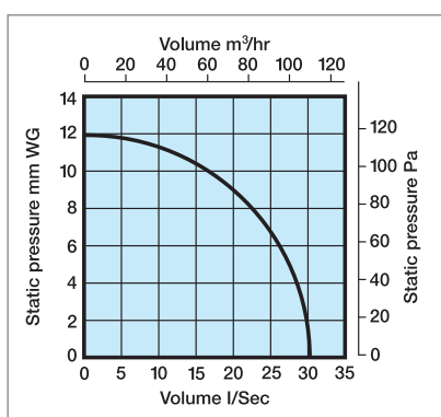
► Performance - EL100
