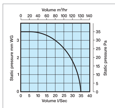
► Performance - EL125
