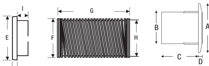
Dimensions - XPLP
